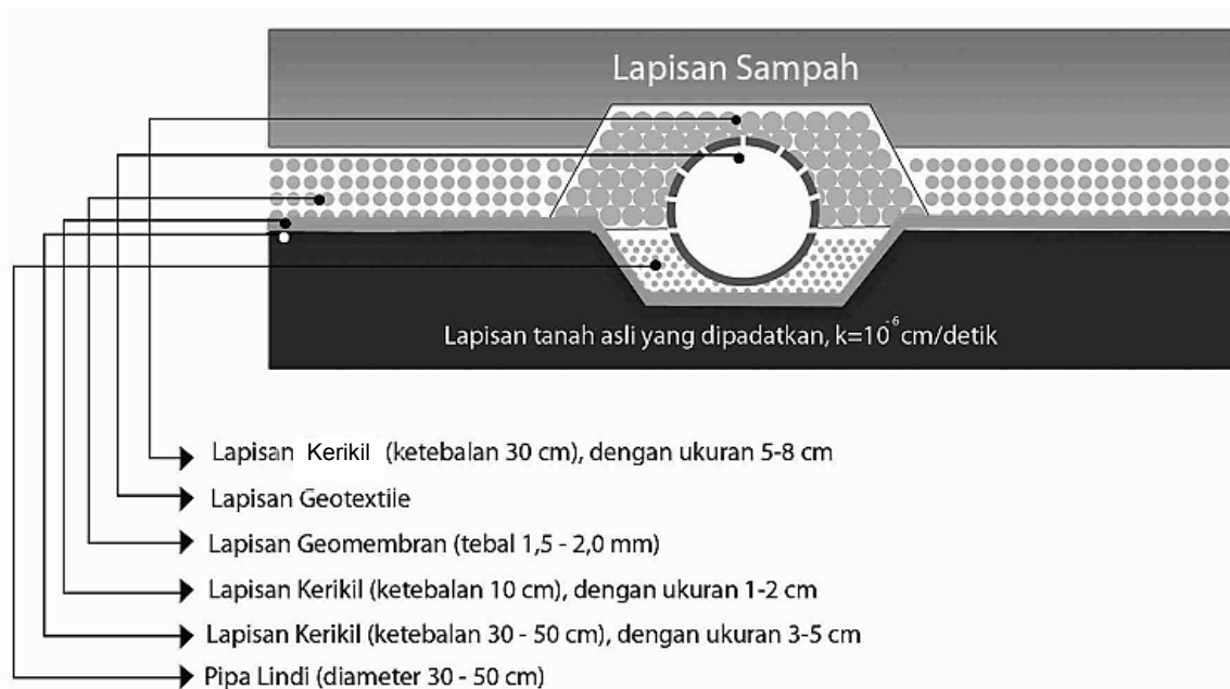
Gambar 7 – Pelapis Dasar Tanah TPA Dengan Geomembran
