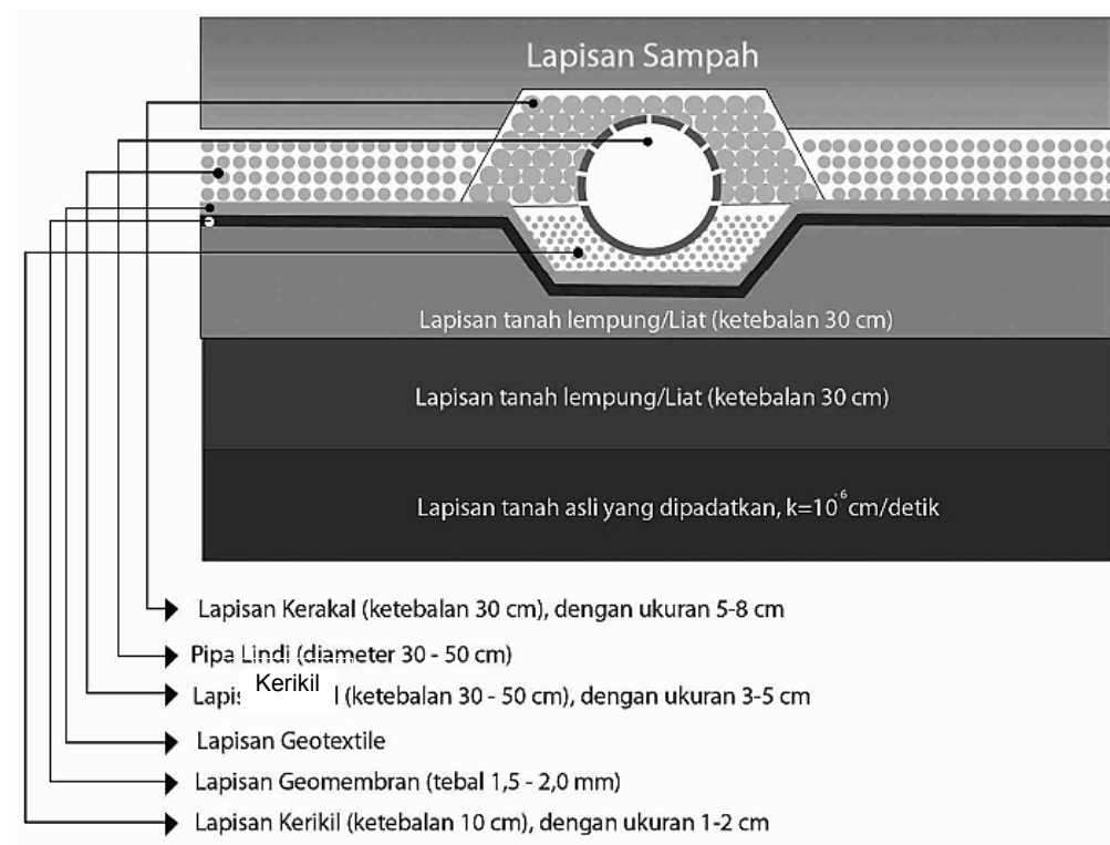
Gambar 6 – Pelapis Dasar Tanah TPA Dengan Geomembran dan Tanah Lempung
