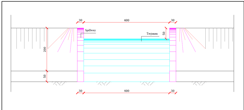
Gambar 4.27. DPn pasangan batu spesi dengan ukuran tinggi = 3 meter dan lebar = 7 meter tampak depan
