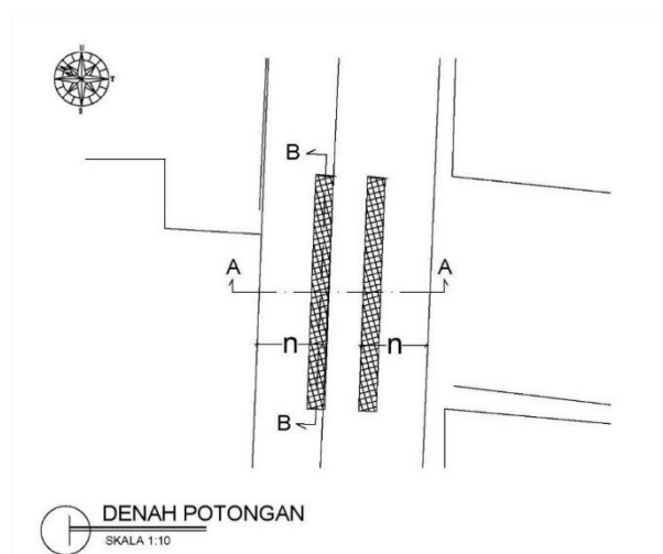
Gambar 4.77. Geoframe Tampak Atas
