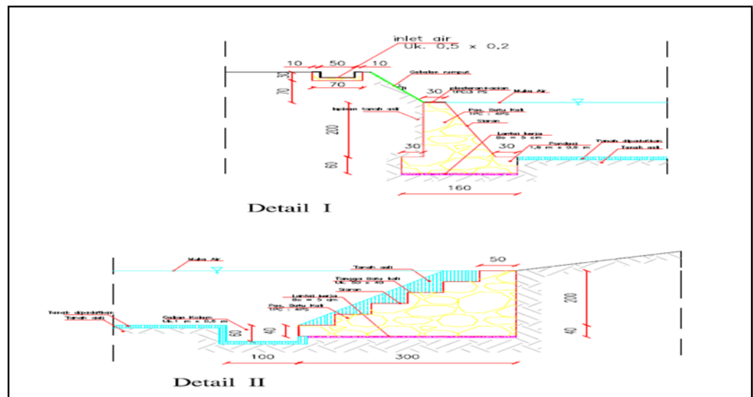
Gambar 4.53. Detail Tangga dan Spillway dari kolam retensi/embung dengan bahan spesi batu
