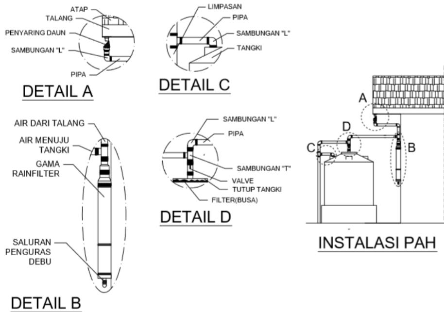
Gambar 4.71. Detail Komponen Rainfilter pada IPAH
