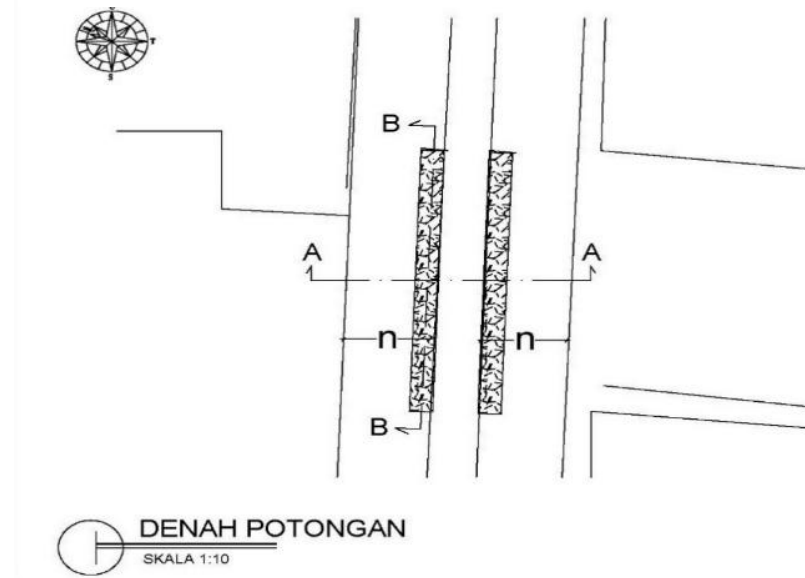
Gambar 4.73. Bronjong Tampak Atas
