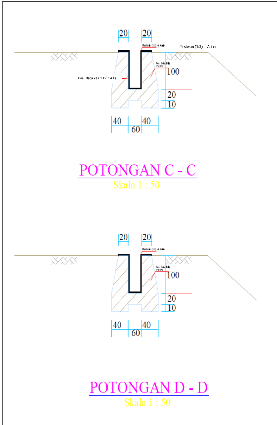
Gambar 4.11. Desain spillway Dam Pengendali tipe urugan tanah komposit
