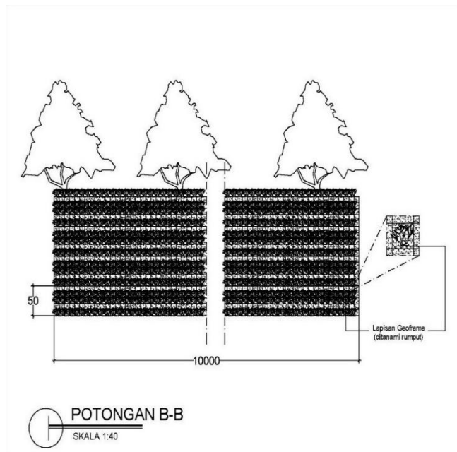
Gambar 4.79. Geoframe Tampak Depan
