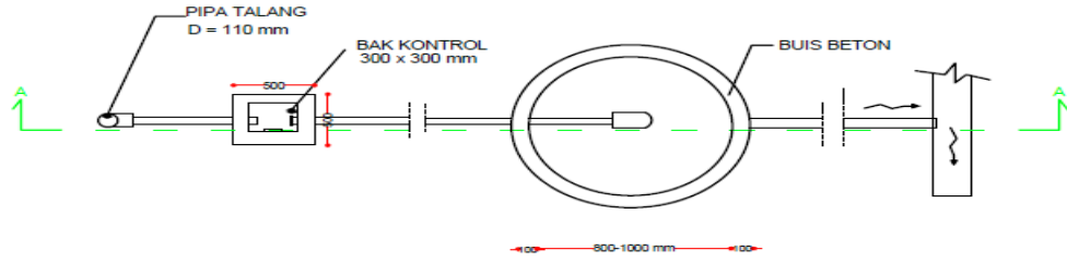
Gambar 4.66. SRA tipe buis beton tampak atas
