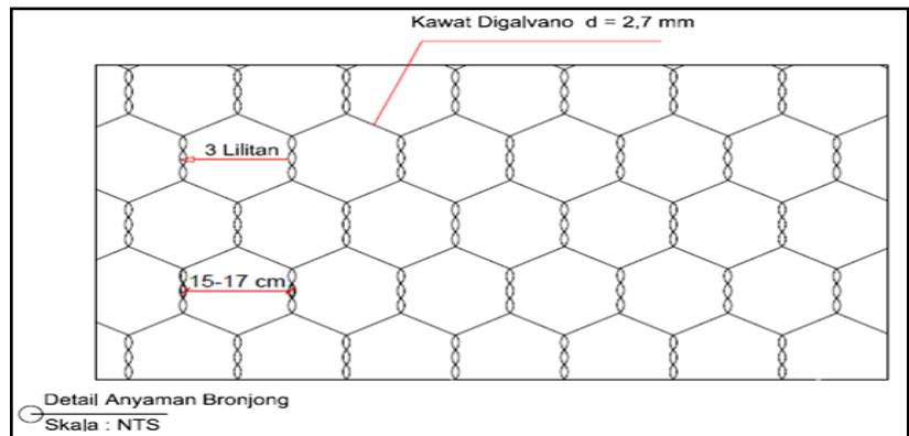
Gambar 4.30. Spesifikasi teknis bronjong DPn
