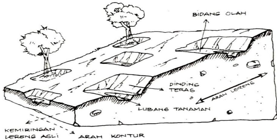
Gambar 4.91. Teras individu
