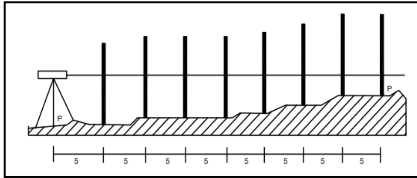
Gambar 6. Profil memanjang
