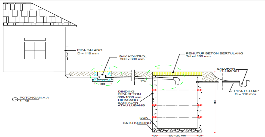
Gambar 8. Desain SRA tipe buis beton
