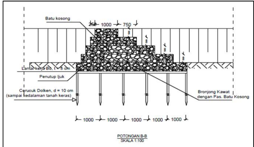
Gambar 4.17. Potongan melintang Dam Penahan Batu Bronjong
