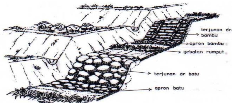
Gambar 4.87. SPA dan Bangunan Terjunan
