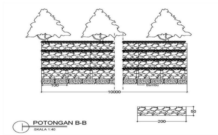
Gambar 4.75. Bronjong Tampak Depan
