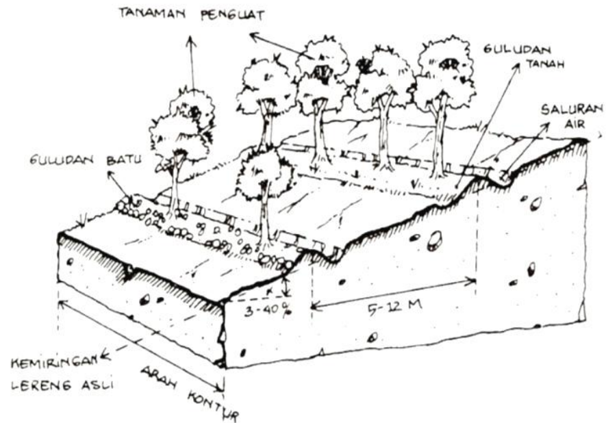
Gambar 4.90. Teras Kredit
