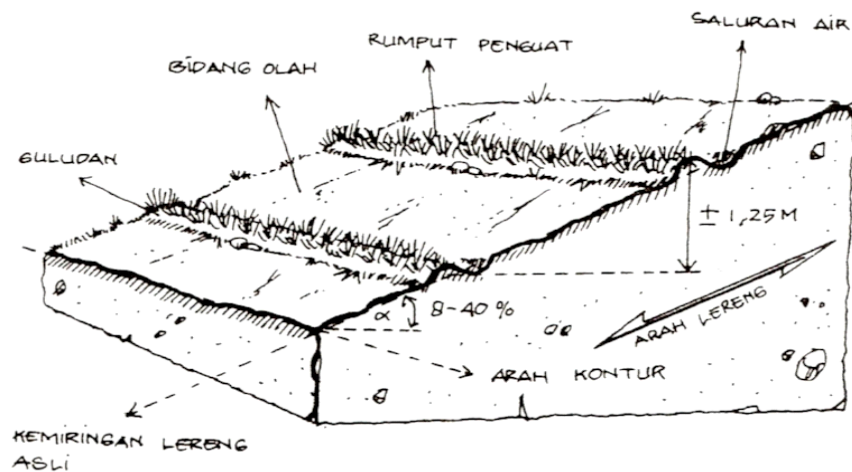
Gambar 4.89. Teras gulud
