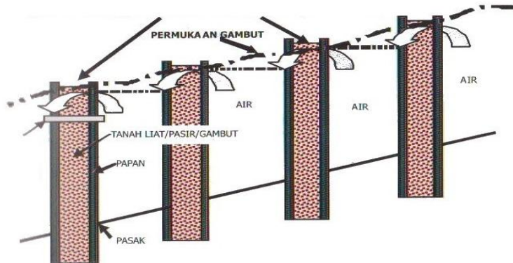
Gambar 8. Letak dan posisi tabat secara melintang
