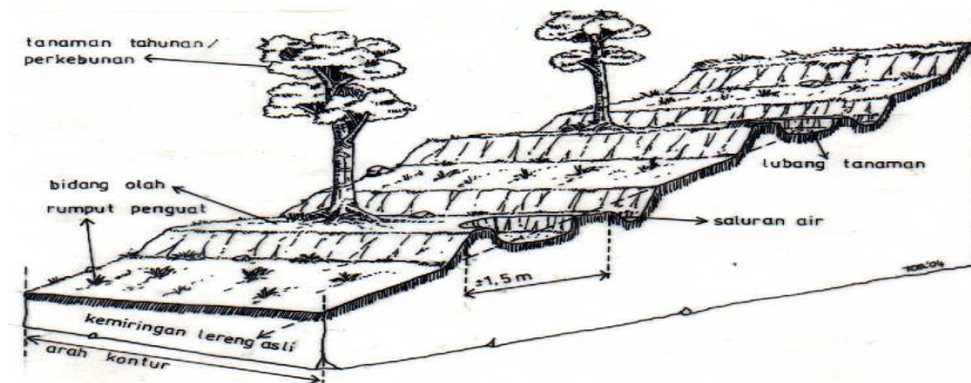
Gambar 4.92. Teras Kebun
