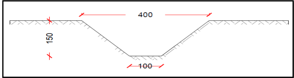
Gambar 4.32. Penampang saluran pengendali jurang tipe batu bronjong
