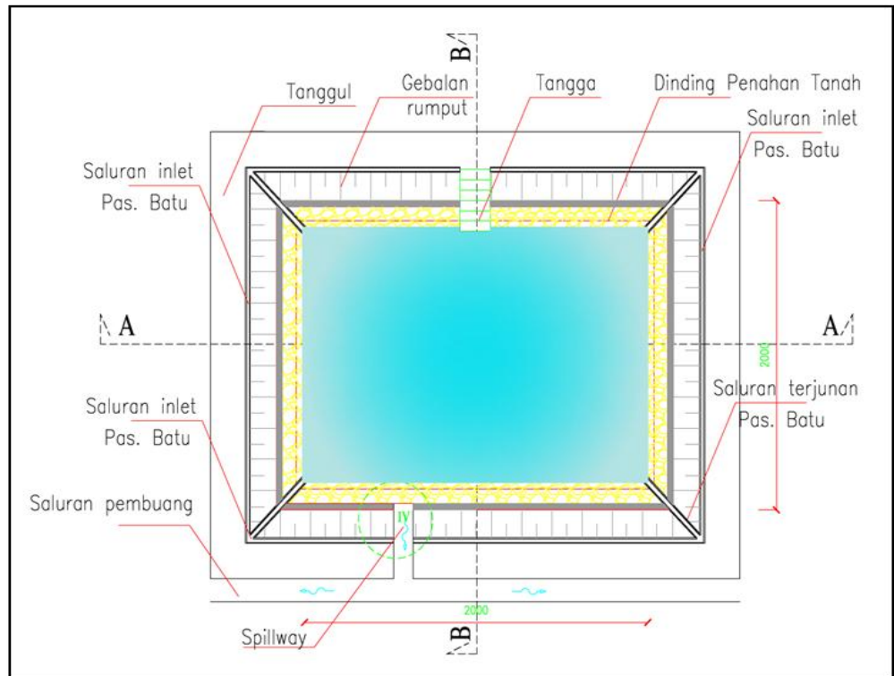
Gambar 4.51. Kolam retensi/embung dengan bahan spesi batu tampak atas
