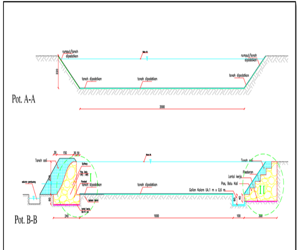
Gambar 4.57. Kolam retensi/embung dengan bahan urugan tanah tampak depan
