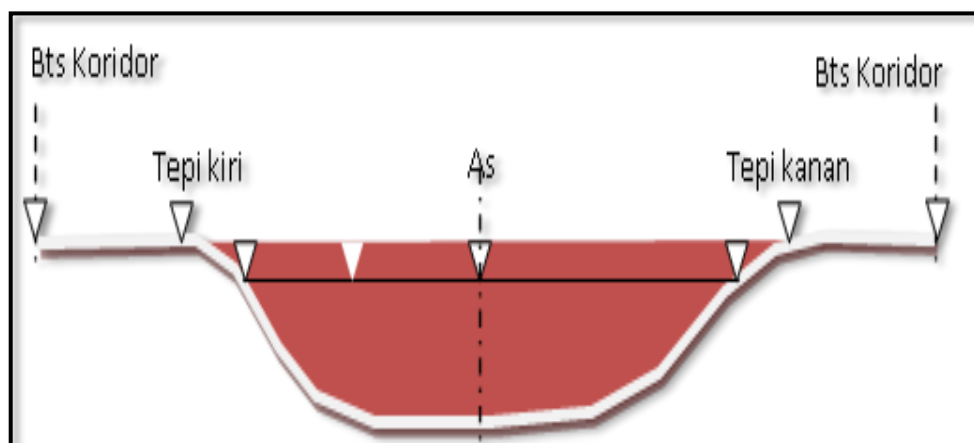
Gambar 7. Profil melintang
