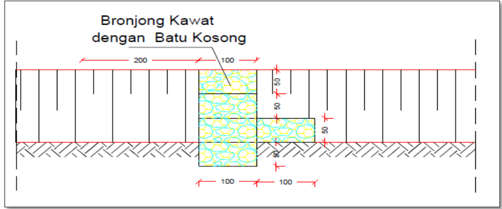
Gambar 4.35. Potongan melintang pengendali jurang tipe batu bronjong
