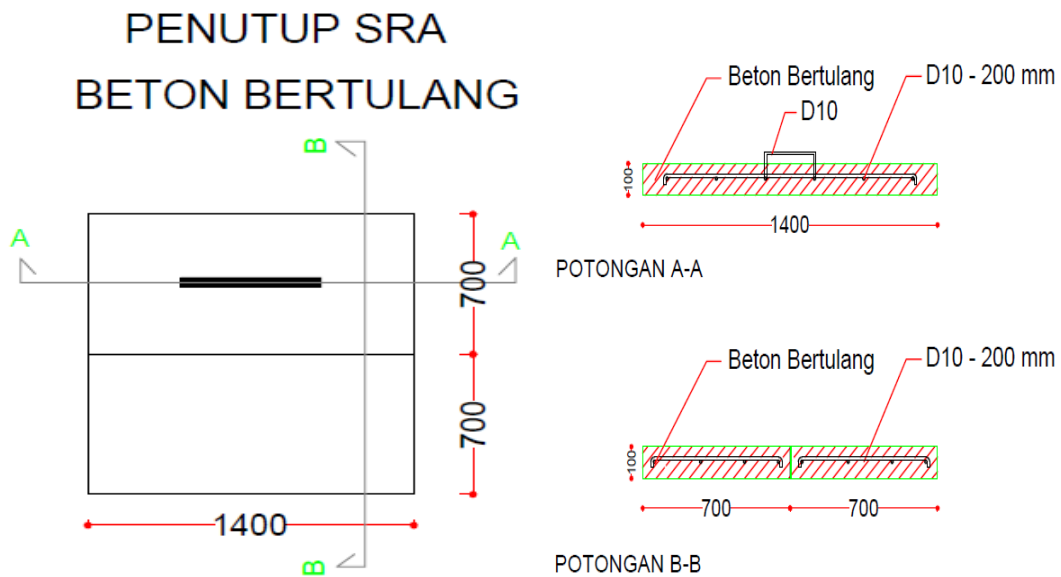
Gambar 4.64. Desain tutup SRA tipe tertutup
