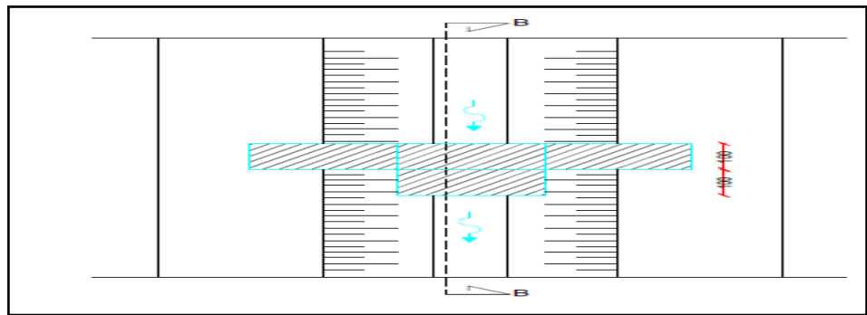
Gambar 4.33. Pengendali jurang tipe batu bronjong tampak atas
