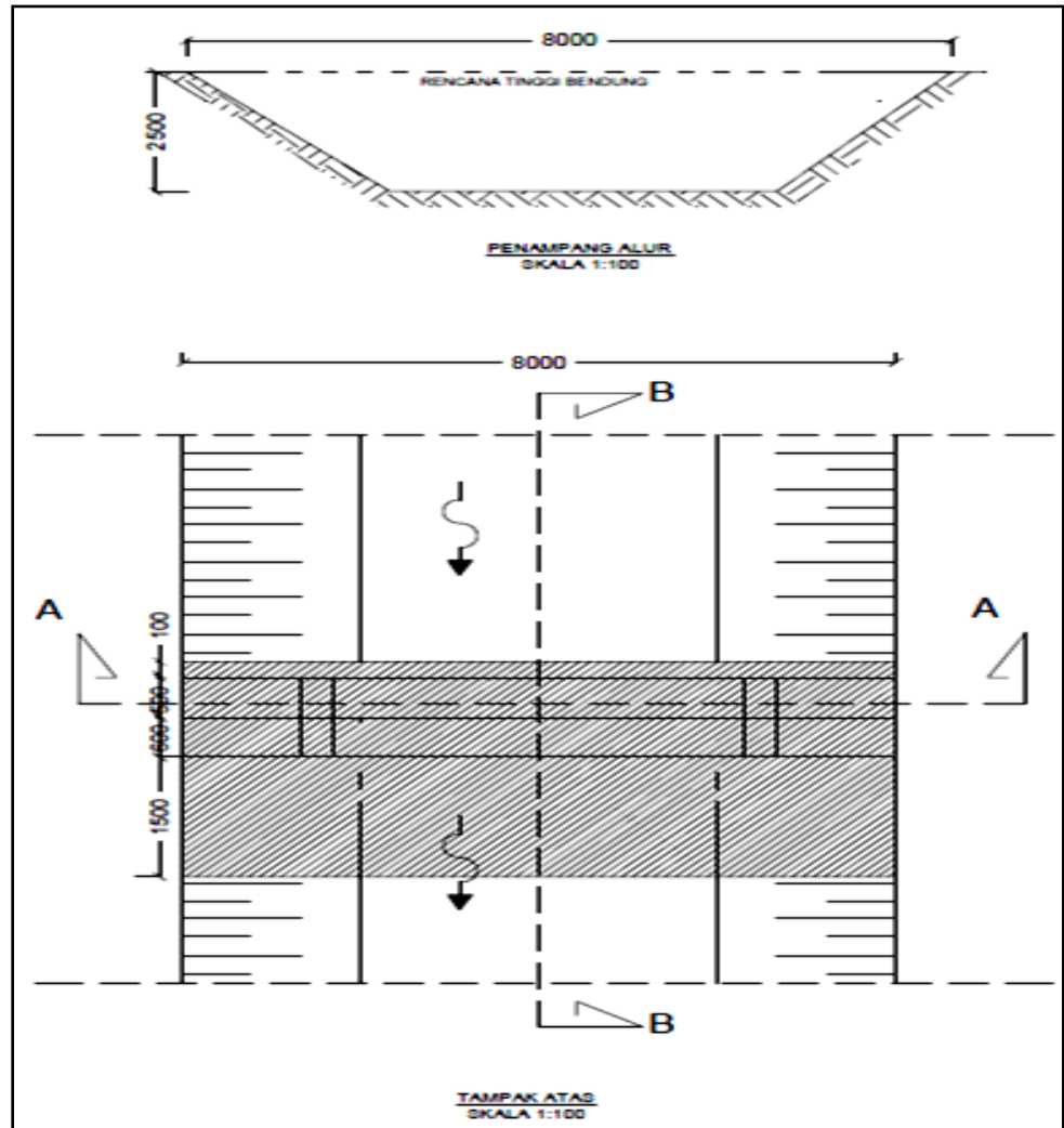
Gambar 4.24. Penampang saluran DPn pasangan batu spesi dengan ukuran tinggi = 3 meter dan lebar = 8 meter
