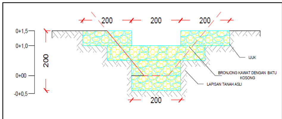
Gambar 4.34. Penampang melintang pengendali jurang tipe batu bronjong
