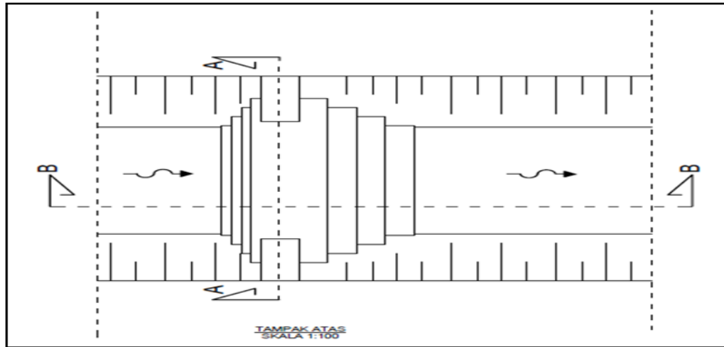
Gambar 4.14. Dam Penahan Batu Bronjong tampak atas
