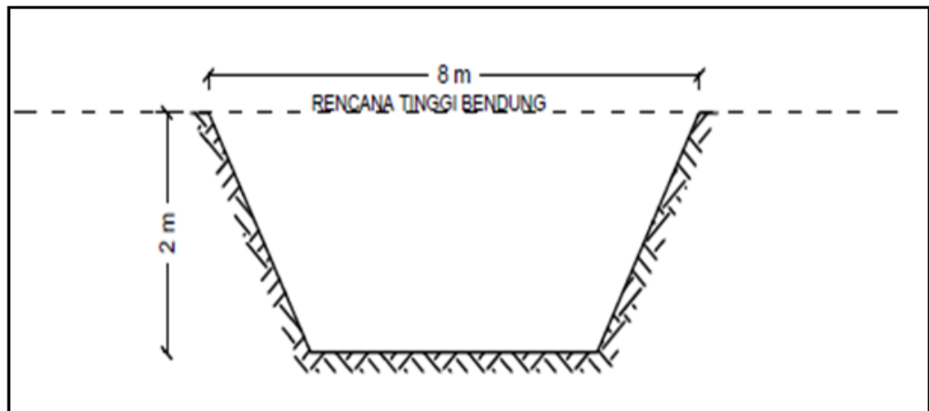
Gambar 4.15. Penampang melintang Dam Penahan Batu Bronjong
