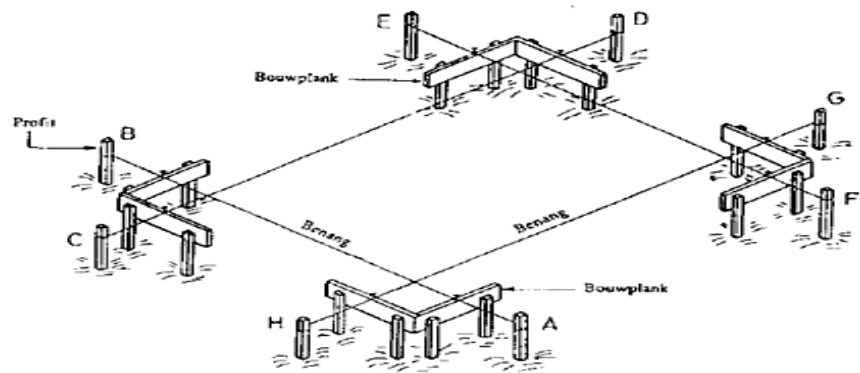
Gambar 4.29. Pemasangan Bouwplank
