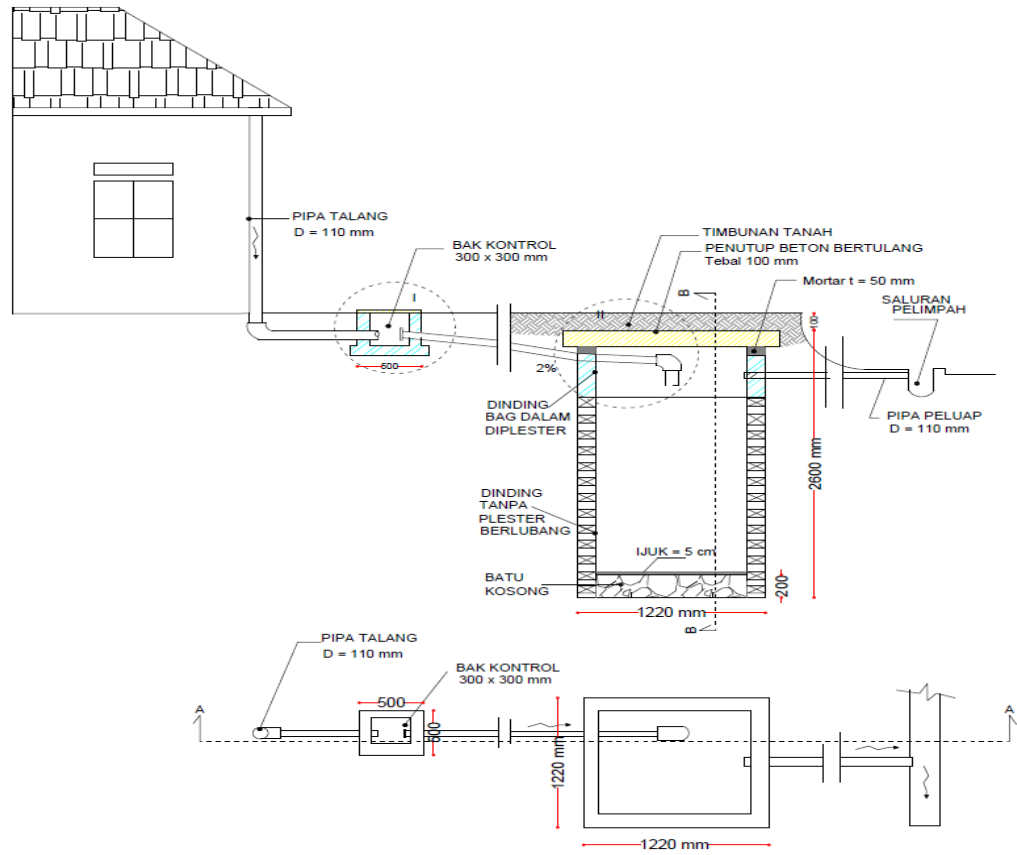
Gambar 4.60. Sumur Resapan Air tipe tertutup
