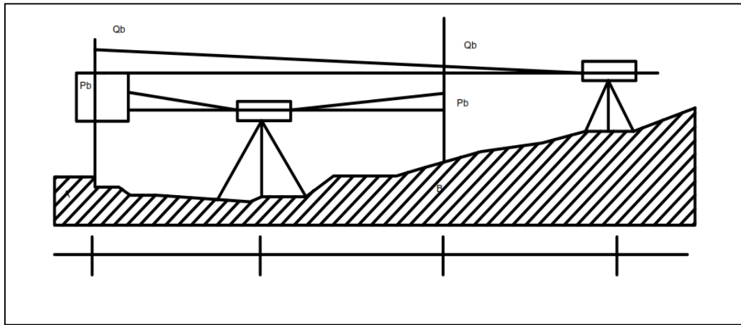
Gambar 2. Pengukuran Beda Tinggi dengan Waterpass
