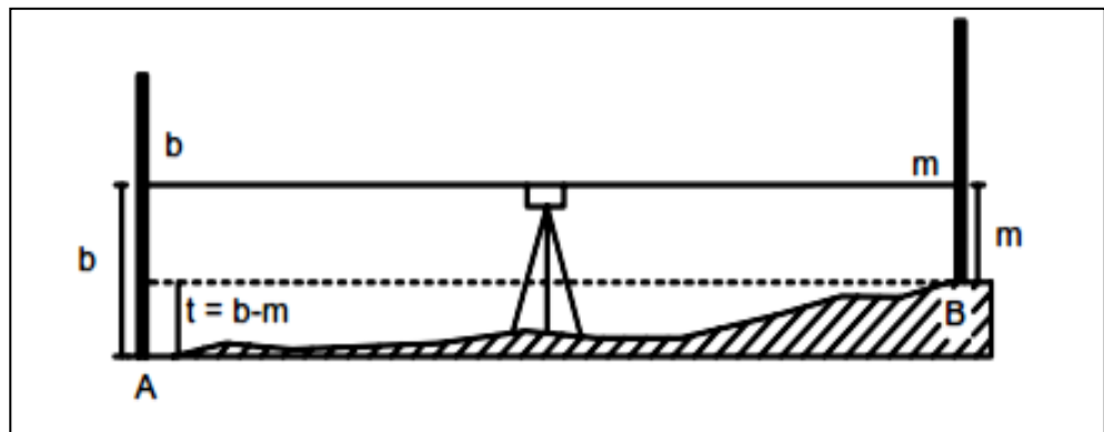
Gambar 4. Pengukuran Beda Tinggi dengan Waterpass (Cara II)
