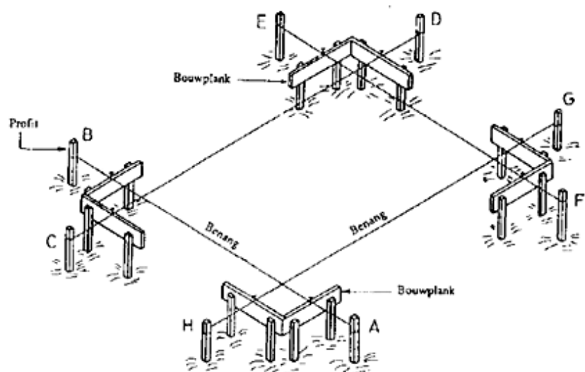
Gambar 4.49. Pemasangan Bouwplank pada bio gully plug
