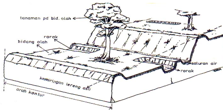
Gambar 4.94. Rorak (saluran buntu)
