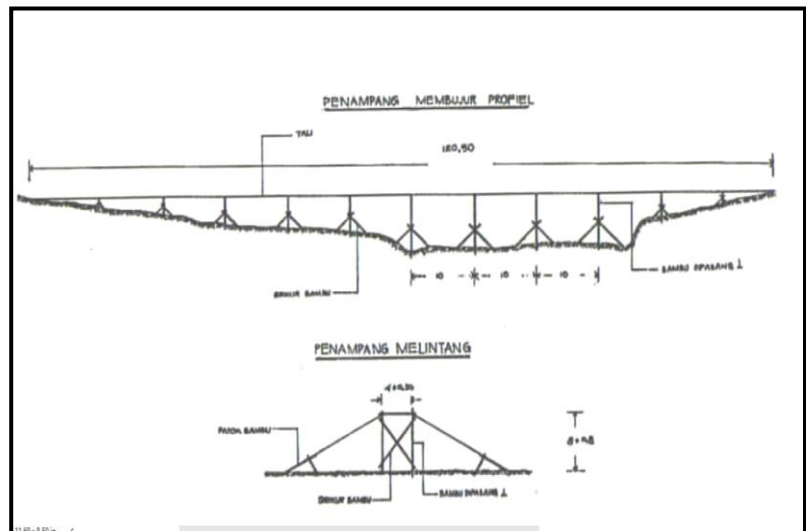
Gambar 4.13. Profil melintang Dam Pengendali
