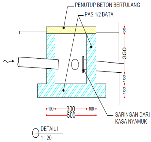
Gambar 4.61. Bak kontrol SRA
