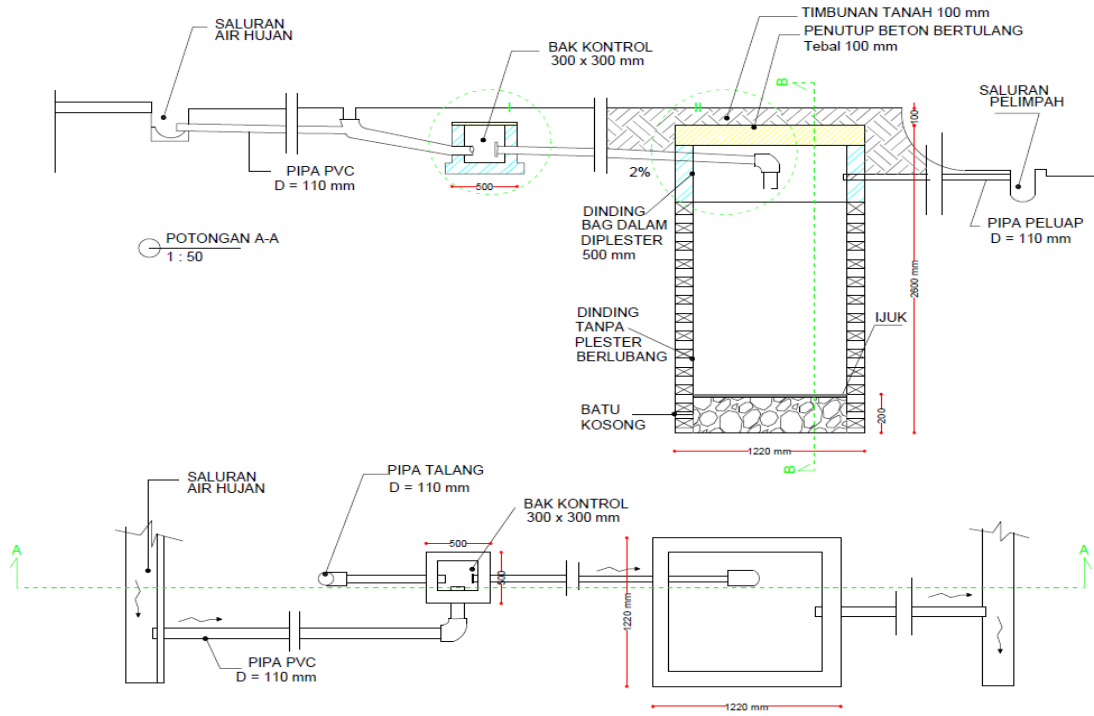
Gambar 4.65. SRA tipe terbuka
