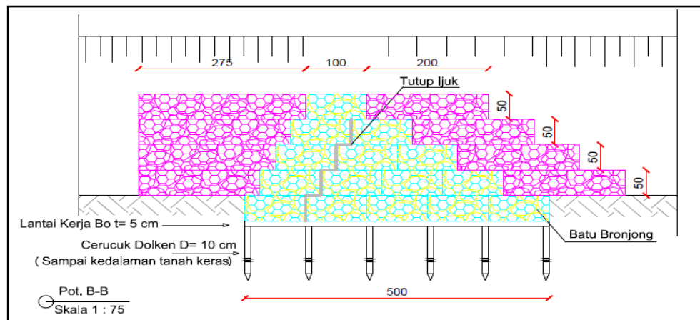
Gambar 4.21. Potongan melintang Dam Penahan Batu Bronjong dengan sayap
