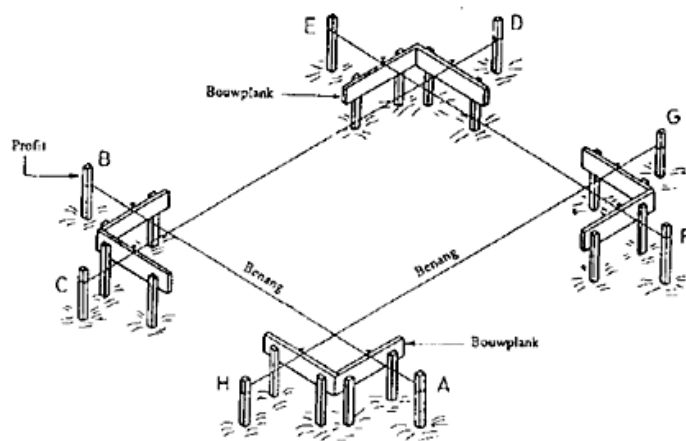
Gambar 4.12. Pemasangan Bouw plank Dam Pengendali
