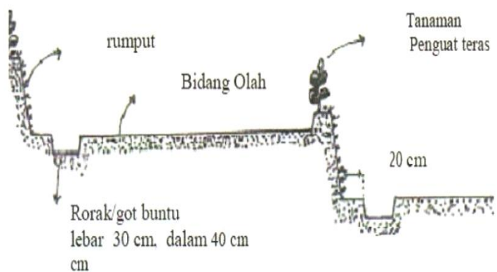
Gambar 4.96. Penampang melintang Rorak (saluran buntu)
