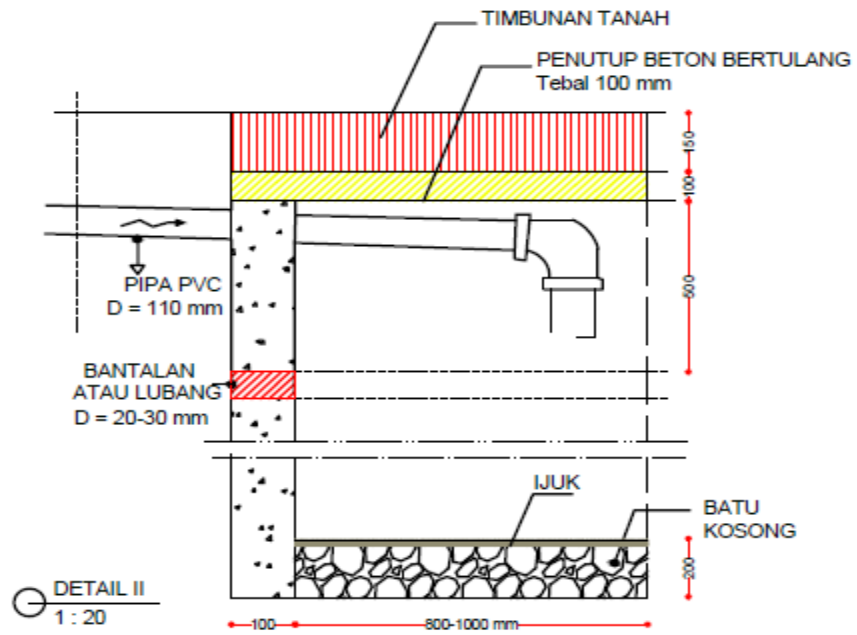
Gambar 4.67. SRA tipe buis beton tampak samping
