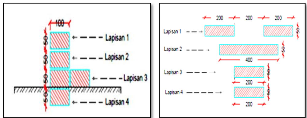
Gambar 4.36. Layout penempatan bronjong
