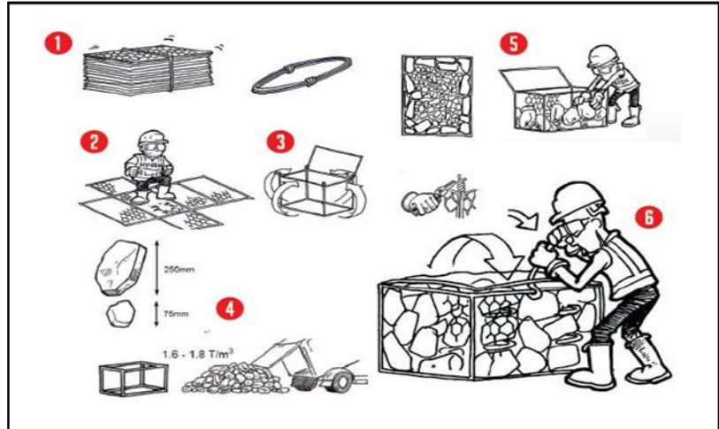
Gambar 4.31. Tata cara pemasangan bronjong
