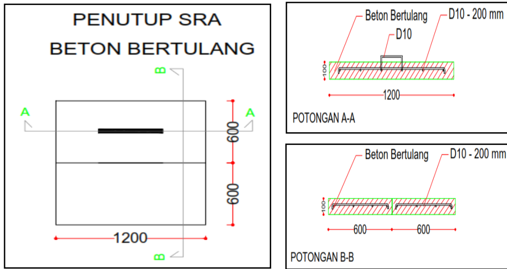
Gambar 4.69. Desain Penutup SRA tipe buis beton
