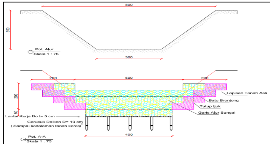
Gambar 4.20. Dam Penahan Batu Bronjong dengan Sayap tampak depan berukuran tinggi =3 meter; Lebar = 8 meter
