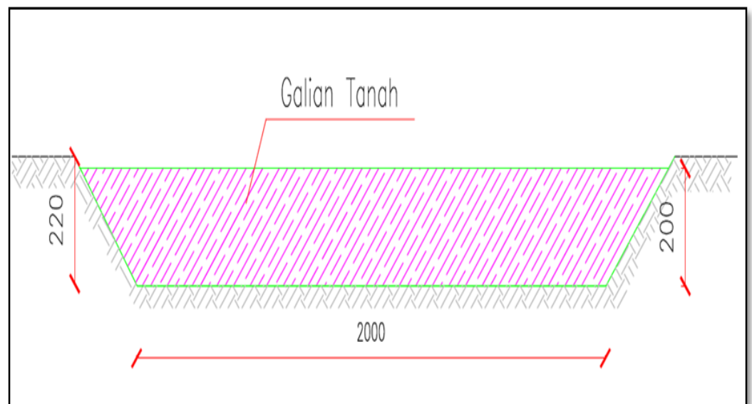
Gambar 4.58. Galian tanah pada kolam retensi/embung dengan bahan urugan tanah
