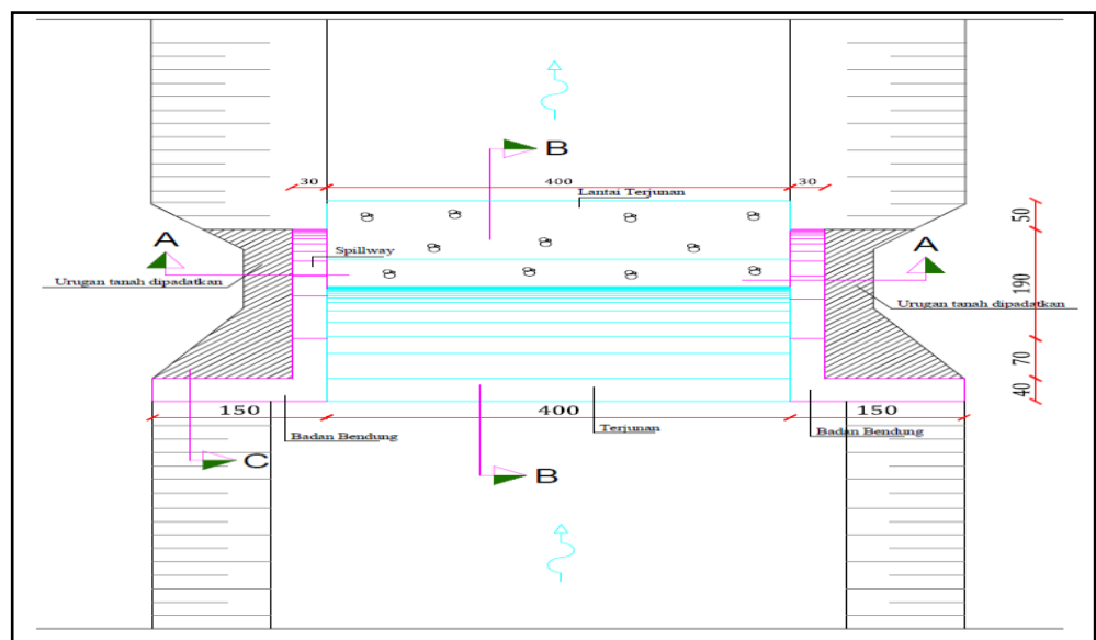
Gambar 4.25. DPn pasangan batu spesi dengan ukuran Tinggi = 3 meter dan Lebar = 7 meter Tampak atas
