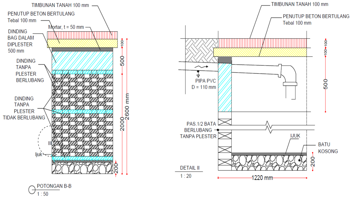
Gambar 4.63. Detil penampang SRA
