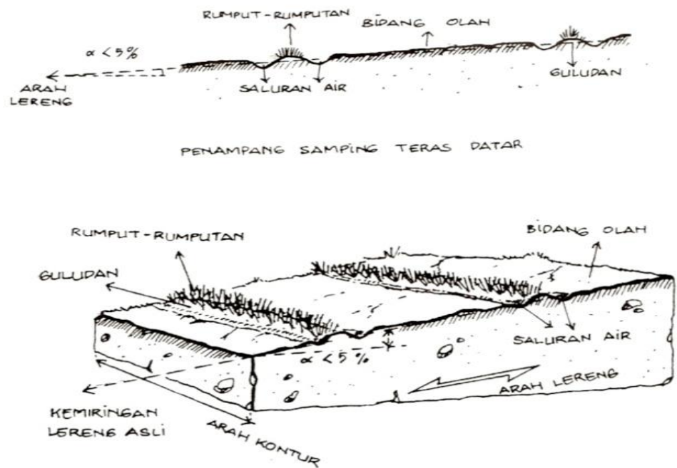
Gambar 4.88.Teras datar
