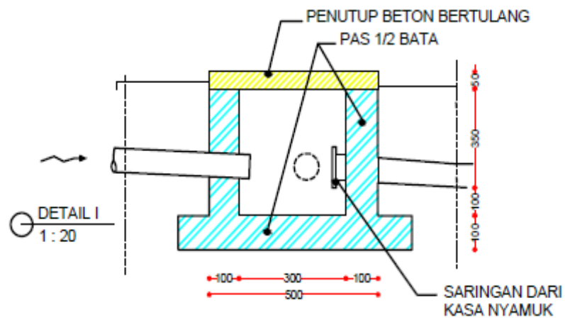
Gambar 4.68. Bak kontrol SRA tipe buis beton
